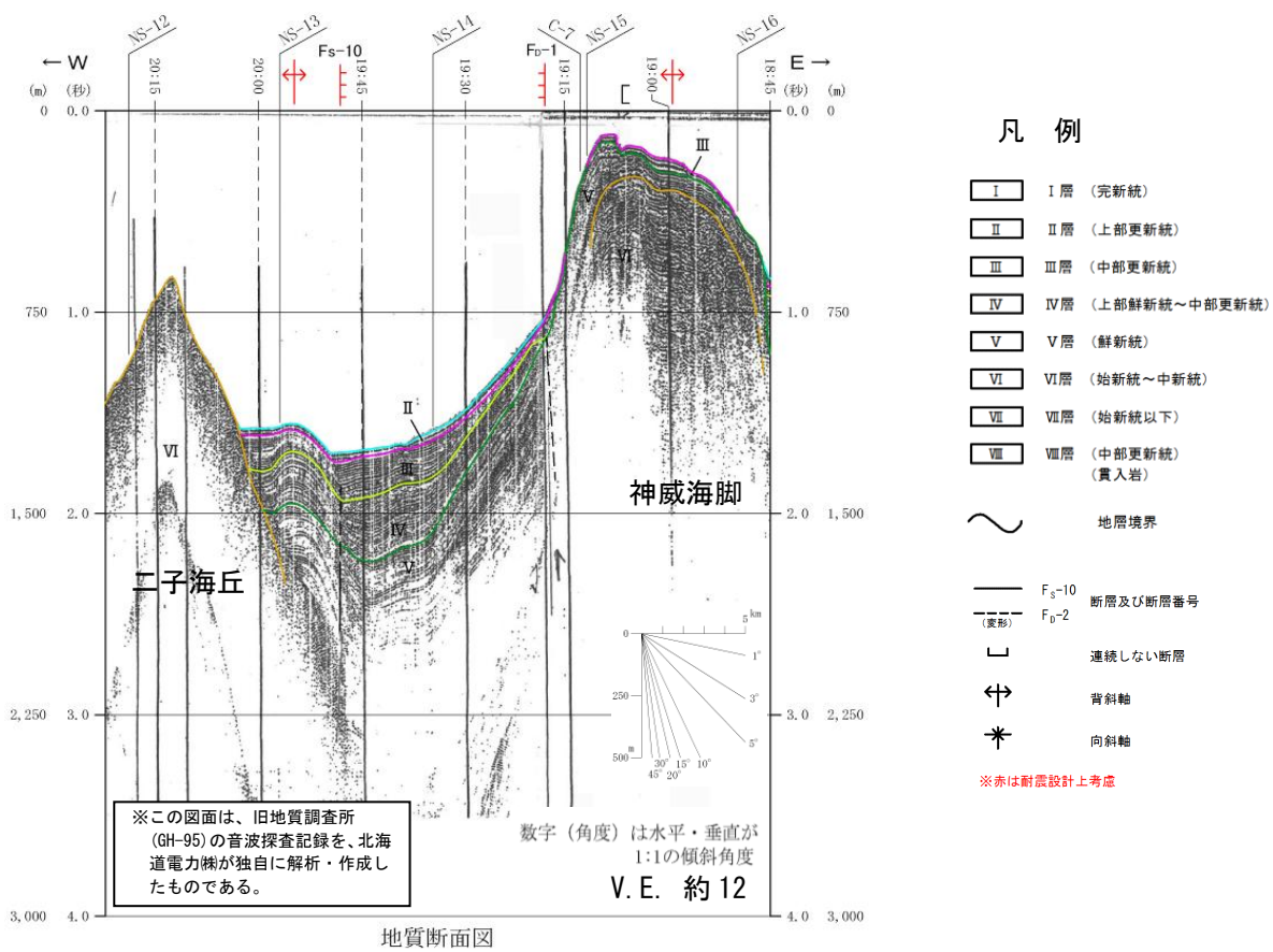
図5 敷地前面海域の音波探査記録（測線 EW-8）
