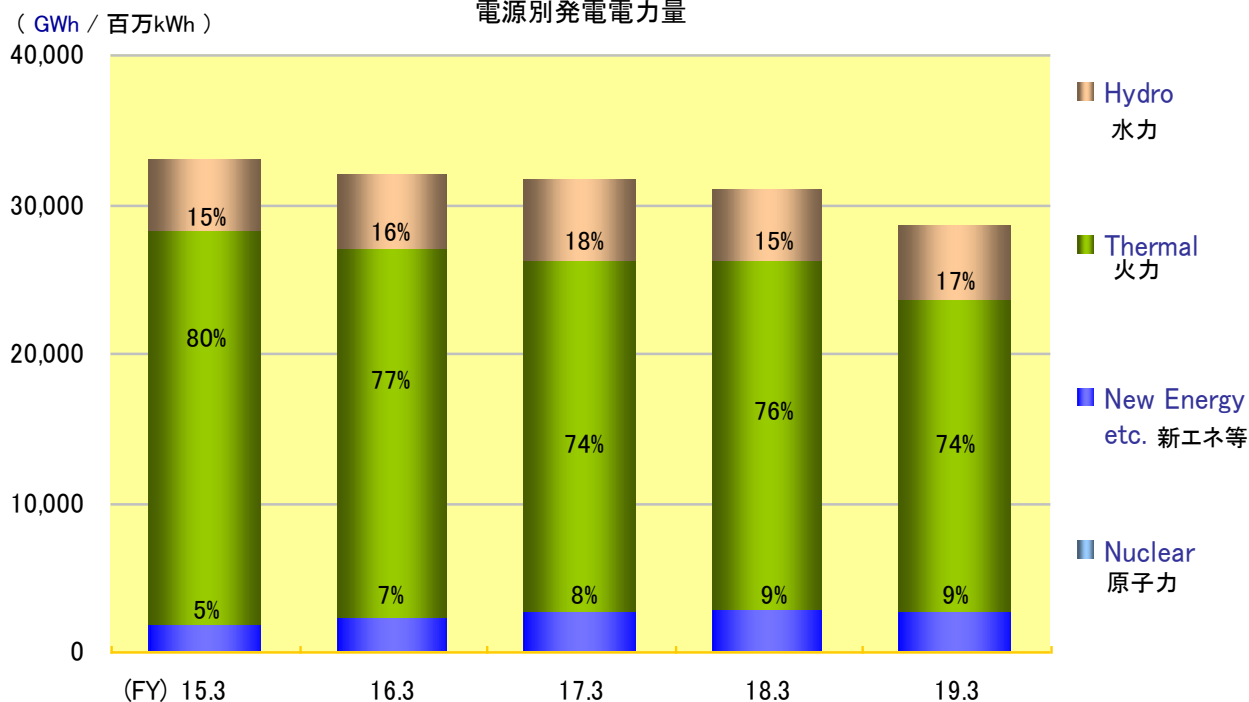
Power Generation by Type 電源別発電電力量
