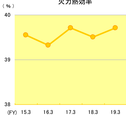
Thermal Efficiency 火力熱効率
