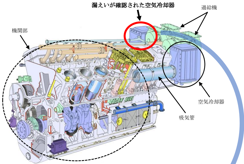
図2：非常用ディーゼル発電機（機関部）鳥瞰図
