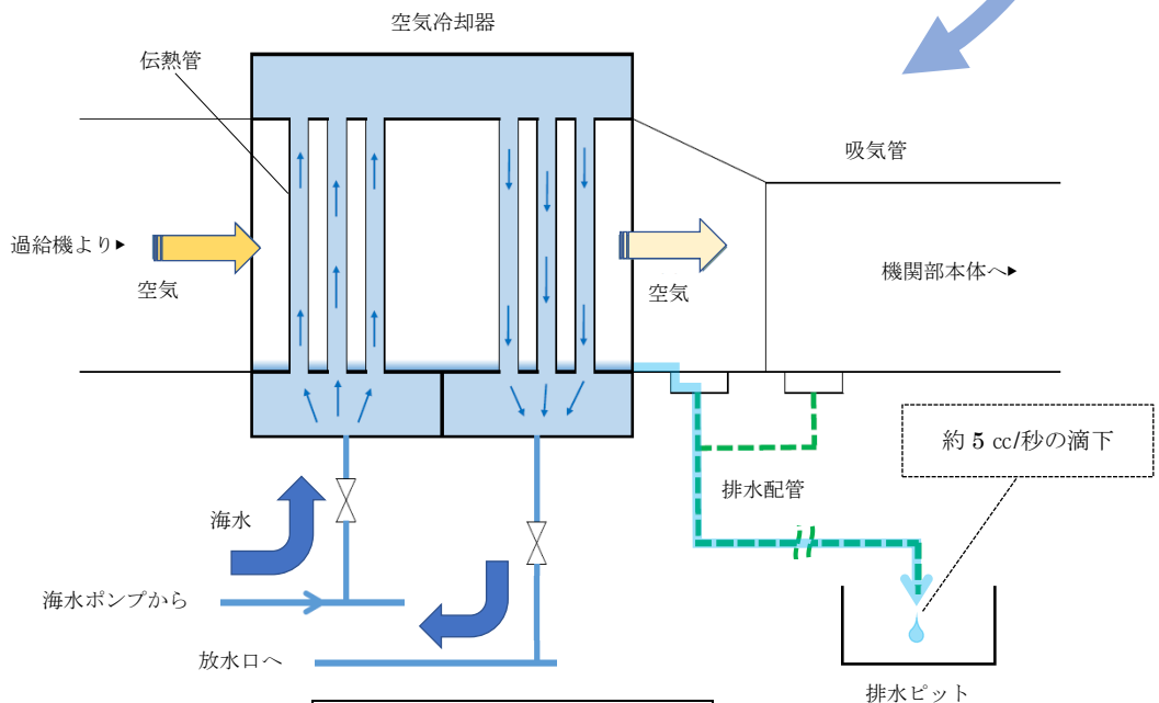
図3：空気冷却器 概略図
